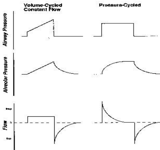
Fig # 3: Comparación de las presiones inspiratorias pico y presión alveolar generadas por las modalidades de flujo constante y decelerante.
