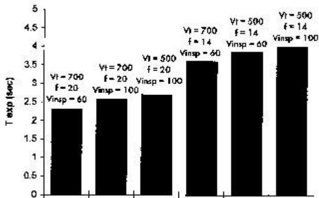
Fig # 2: Comparación del efecto del incremento del flujo inspiratorio ( V_{insp} ), la disminución del volumen tidal ( V_t ) y la disminución de la frecuencia respiratoria ( f ), sobre el tiempo espiratorio.
